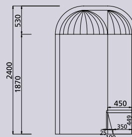
PRESJEK B-B
