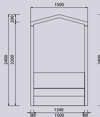
PRESJEK A-A
