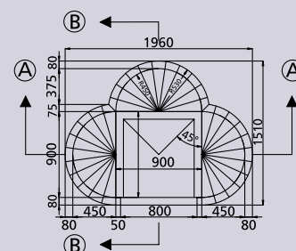
TLOCRT
