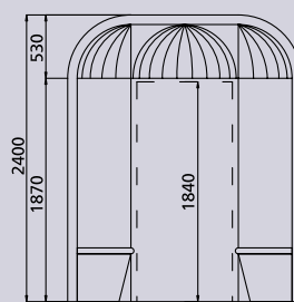
PRESJEK A-A
