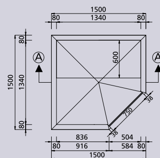
TLOCRT
